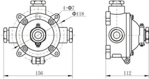
Pendant type lighting terminal box
